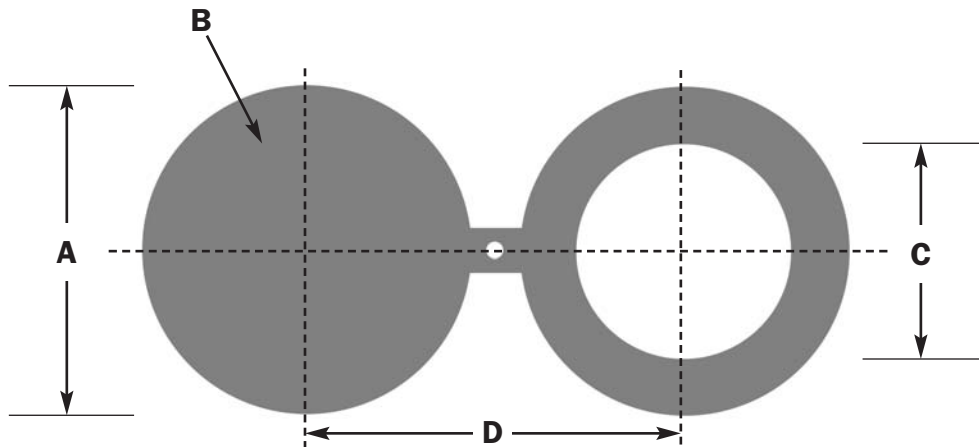
Spectacle Blind
