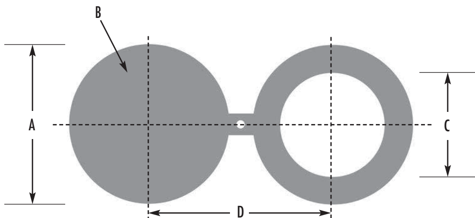
Spectacle Blind
